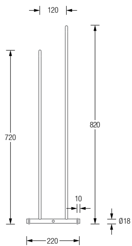
HTB2K-500 / 700 Seitenansicht:
