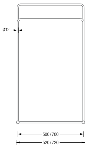
HTB2K-500 / 700 Frontansicht:
