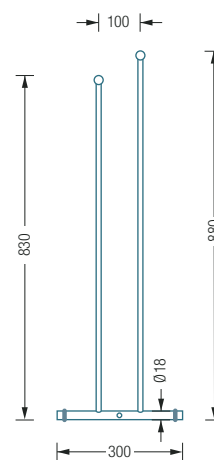
HTB2 Seitenansicht:
