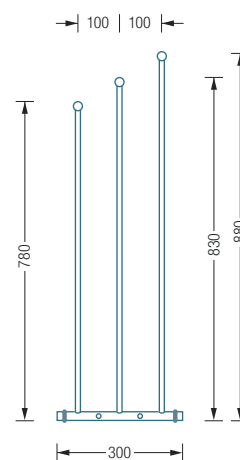
HTB3 Seitenansicht:
