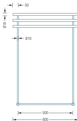
HTB3 Frontansicht:
