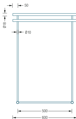
HTB2 Frontansicht:
