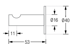
HV16-50R40-B Seitenansicht:
