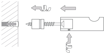
Montage HV16-50-B:
