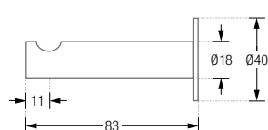
HV18-80R40-B Seitenansicht:
