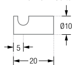
HV10-20-B Seitenansicht:
