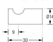
HV14-30K40-B Seitenansicht:
