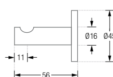
HV16-50K45-B Seitenansicht:
