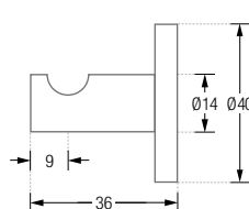
HV14-30K40-B Seitenansicht:
