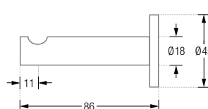
HV18-80K45-B Seitenansicht:
