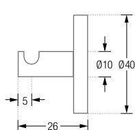
HV10-20K40-B Seitenansicht:
