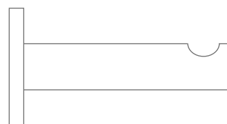
HV18-80K45 Ø18 mm zur Verklebung, Länge 86 mm.
