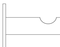
HV16-50R40 Ø16 mm zur Verschraubung, Länge 53 mm.
