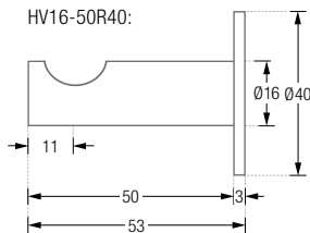
HV16-50R40:
