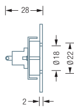
KK50 Seitenansicht:
