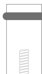
MG015-30 mit O-Ring zur rückseitigen M4-Senkkopf-Verschraubung
