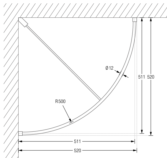
Produktbeispiel G500VW Draufsicht:
