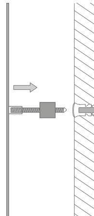
Montage BFSS-Set2 mit optional verwendbaren Wandabstandshülsen:
