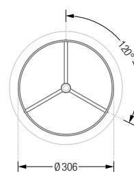
GSST Draufsicht:
