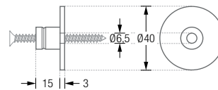
R40H Seitenansicht / Draufsicht:
