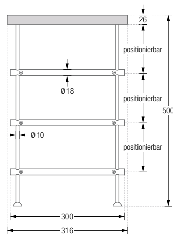
Produktbeispiel SB800-3-Eiche-B Seitenansicht:
