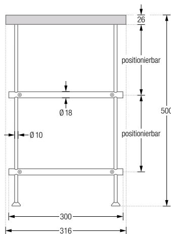
Produktbeispiel SB800-2-Eiche-B Seitenansicht:
