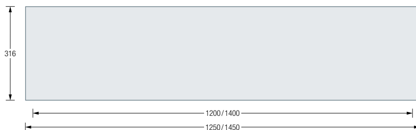
SBS1200-4-Eiche / 1200-5-Eiche / 1400-4-Eiche / 1400-5-Eiche Draufsicht:
