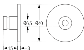
R40H Seitenansicht/Draufsicht:
