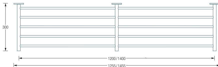
SR1200-1W / 1400-1W Draufsicht:
