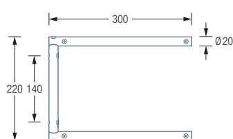
SR600-2W / 700-2W / 800-2W / 900-2W / 1000-2W Seitenansicht:
