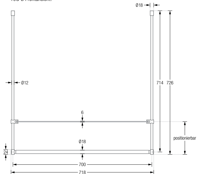
TOG-B Frontansicht:
