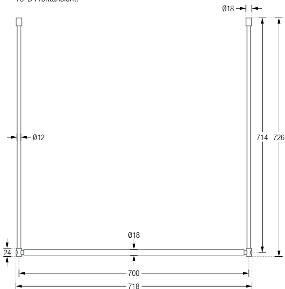
T0-B Frontansicht:
