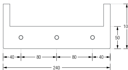
TG3 Frontansicht:
