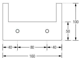
TG2 Frontansicht:
