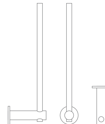
RTPH2-260D Seitenansicht/Frontansicht/Draufsicht:
