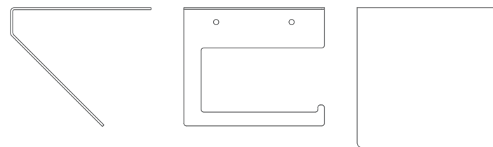
TPHS Seitenansicht/Frontansicht/Draufsicht:
