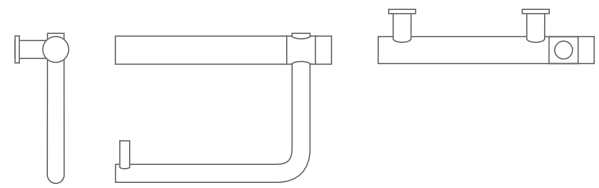
TPH4 Seitenansicht/Frontansicht/Draufsicht:
