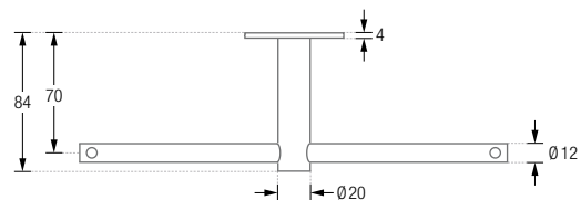
TPH3-260D Draufsicht:
