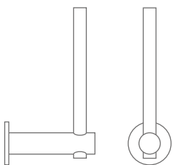
RTPH2-140 Reserverollenhalter zur Verschraubung
