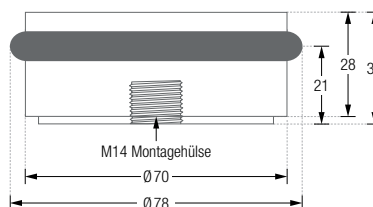
TSB70-30V:
