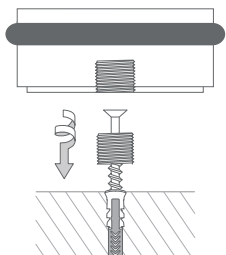
Montage TSB70-30V:
